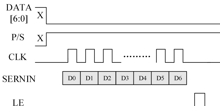
串联控制时序图
