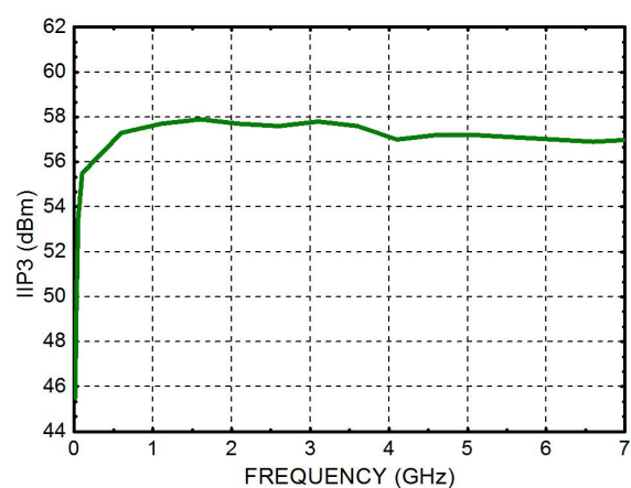
IIP3
