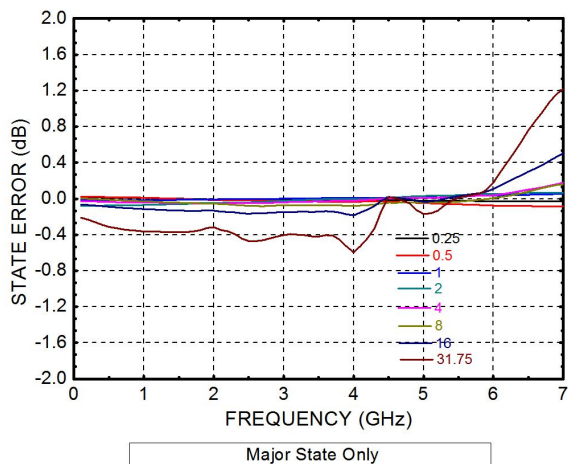
衰减误差
