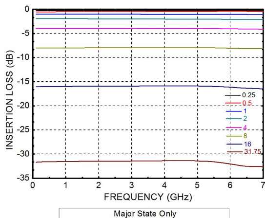
衰减量
