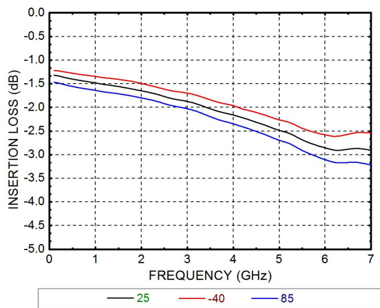
插损 vs. 温度
