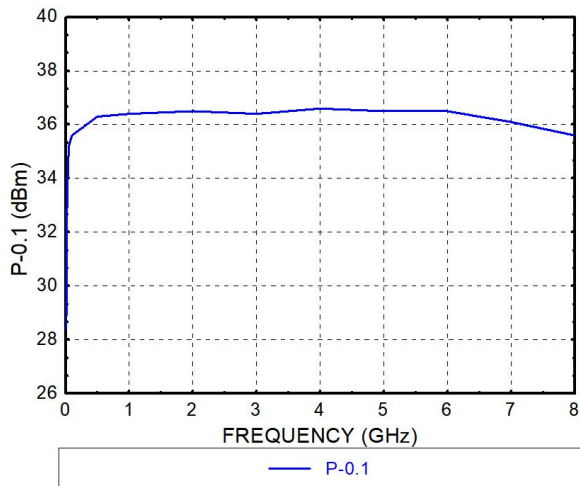
输入 P_{-0.1} (10MHz~7GHz)
