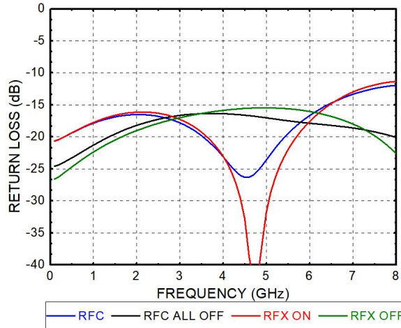
回波损耗
