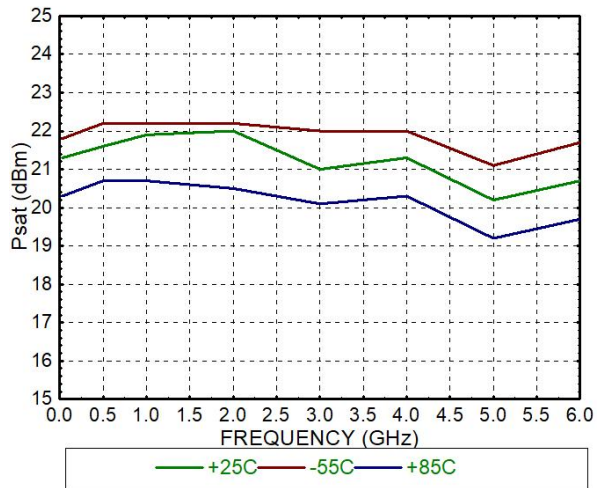
Psat@VG悬空
