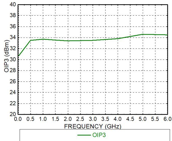
OIP3@VG悬空
