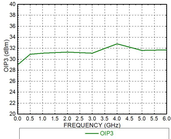
OIP3@VG接地
