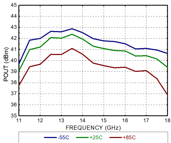
输出功率 VS 温度 (Pin = +24dBm)
