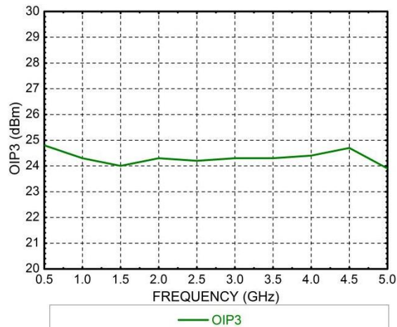
OIP3@VG接地
