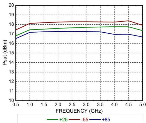
Psat@VG悬空
