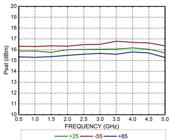
Psat@VG接地
