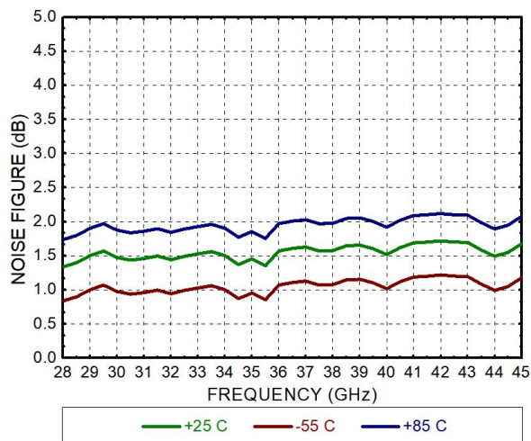
噪声系数
