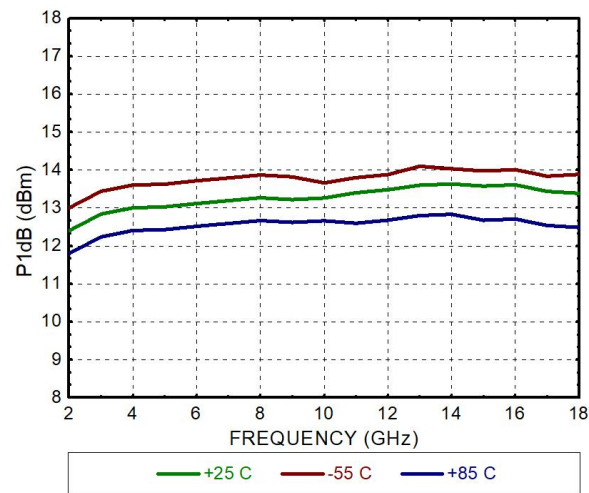
输出功率 P_{1\text{dB}} @VG悬空
