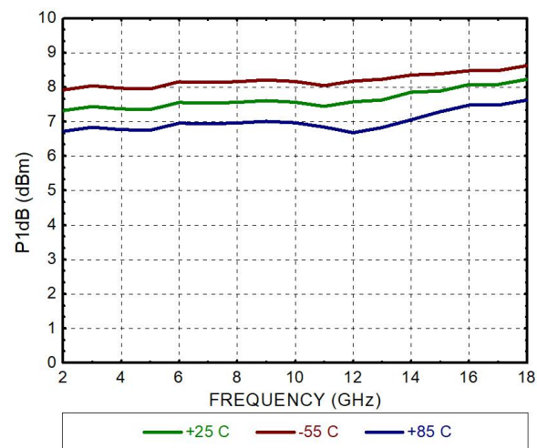
输出功率 P_{1\text{dB}} @VG接地
