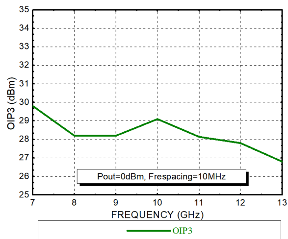
OIP3
