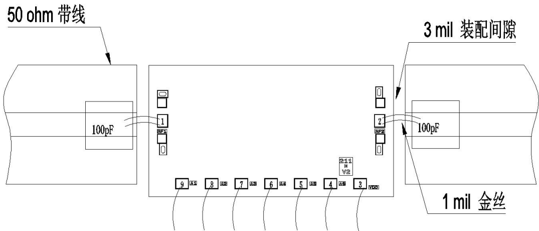
推荐装配图
